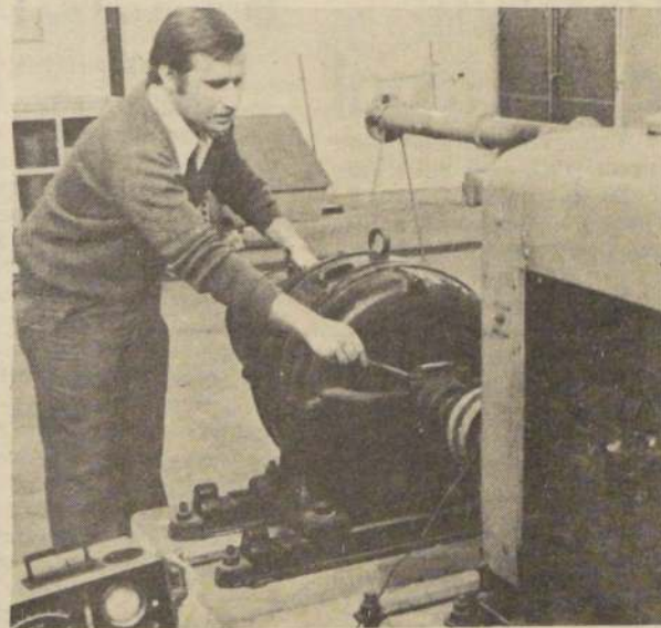
EL INGENIERO Jorge Ramírez muestra un motor que fue acoplado a un dinamómetro para medir la potencia de la mezcla gasolina-metanol.
