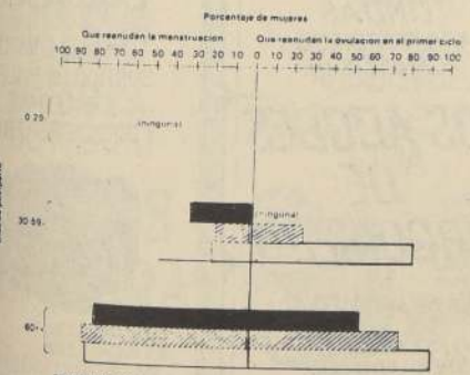
Fig. 2 Porcentaje de mujeres que reanudan la menstruación y la ovulación en el primer ciclo por número de días después del parto y el estado de amamantamiento al tiempo de la primera hemorragia.
