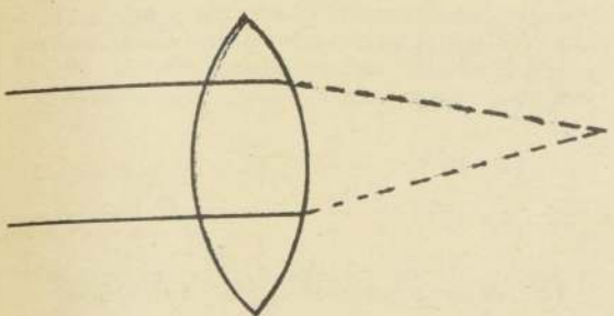
Esquema que demuestra el poder de convergencia de una lente biconvexa.
