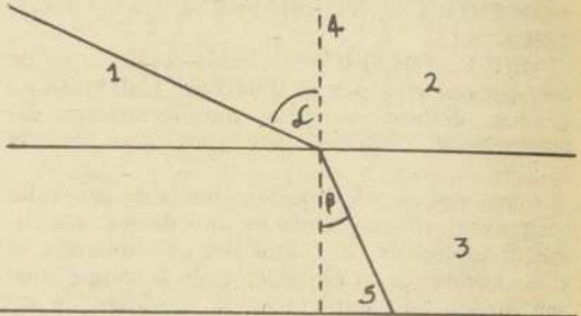
Ejemplo de refracción.
