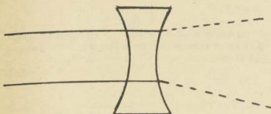
Esquema que demuestra el poder de divergencia de una lente biconcava
