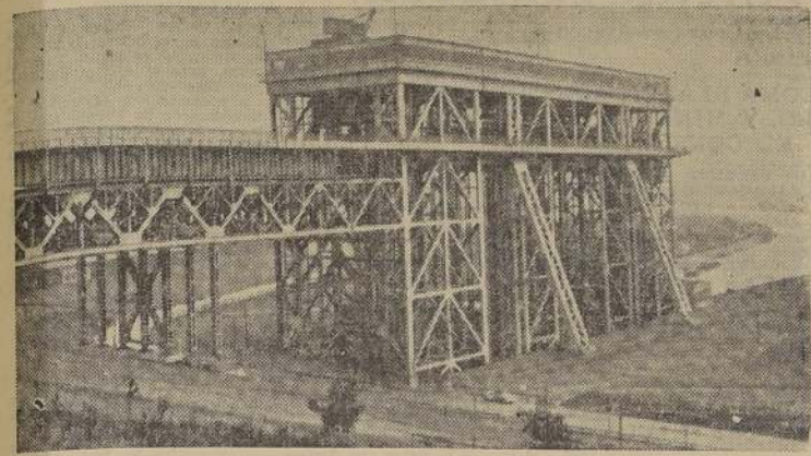
El elevador de vapores nivela una diferencia de altura de 36 metros
