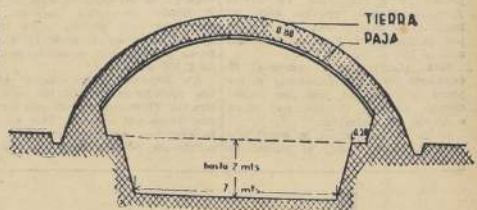
CORTE LONGITUDINAL DE UN SILO ZANJA
