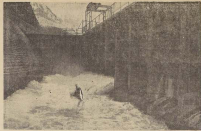
TALCA. BOCATOMA ARMERILLO DEL SISTEMA MAULE NORTE.— 250 kilómetros en canales comprende el Sistema de Riego Maule Norte, de los cuales están terminados ya cerca del 45%, y que con el Embalse Digua permitirán el riego total de las provincias de Linares y Talca. Ambas obras las realiza el Ministerio de Obras Públicas, dentro de la Alianza para el Progreso. En el grabado, una vista de la bocatoma Armerillo del Sistema Maule Norte.
