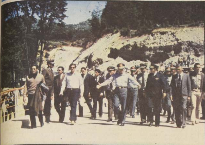
EL PRESIDENTE DE LA REPUBLICA y comitiva recorren el puente "El Espolón", durante la inauguración del camino de Futaleufú a Puerto Ramírez, que empalmará con la Carretera Austral. El puente tiene una longitud de 80 metros y 6,10 de calzada y fue realizado en hormigón armado y superestructura de viga metálica con losa colaborante.
