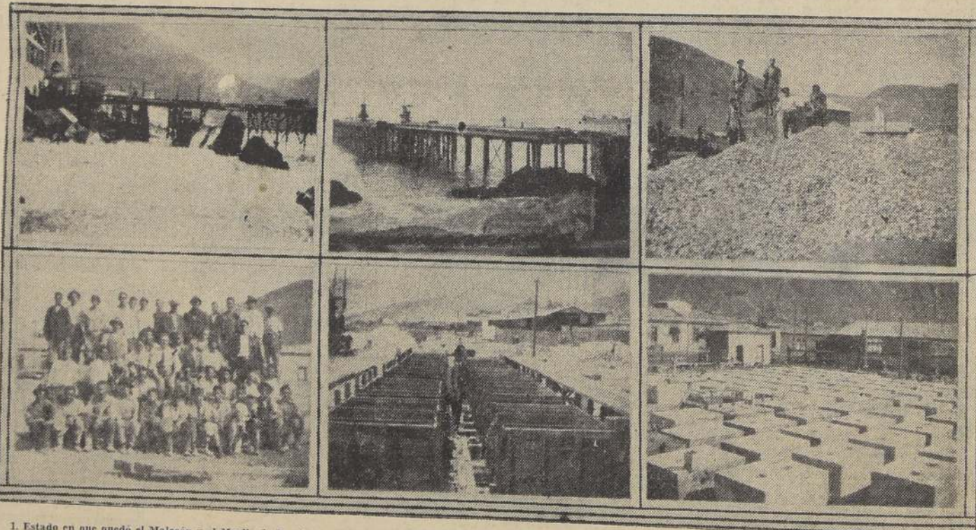
1. Estado en que quedó el Malecón y el Muelle de Pasajeros, que será abandonado. — 2. El Muelle Fiscal, que será reparado y habilitado para el desembarco de pasajeros y pacotilla. — 3. Recopilación de ripio. — 4. Personal que se ocupa en los trabajos. (El marcado con X es el señor López, Conductor de Obras). — 5. Cajones para la hechura de los blocks de concreto. — 6. Parte de los blocks ya hechos.
