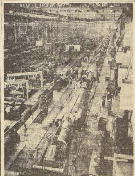
LA LINEA DE CONFORMACION DEL LOCKHEED F-104. — Las secciones del fuselaje del avión ultrasonico "F104 Starfighter", forman largas filas, hasta donde la vista alcanza, en los talleres de montaje de la División de California, de la Lockheed Aircraft Corporation, en Burbank. Después de ajustarse las secciones de los fuselajes, estos se remolcan hasta las plantas de Palmdale, para su ensamblaje final y las oportunas pruebas de vuelo.
