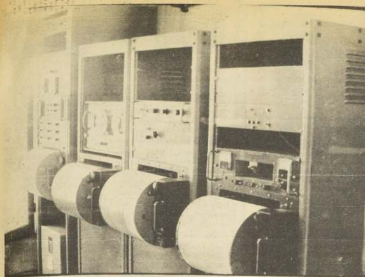
Estos cuatro sismógrafos, conectados con los sismómetros colocados en el subterráneo del movimiento de tierra en Santiago y sus alrededores. Uno de ellos recibe directamente desde la estación de Longaví, a través de Entel.
