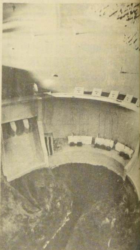
Una perfecta réplica a escala de la Central Hidroeléctrica Rapel, la segunda del país. Genera 350.000 kilowatts.
