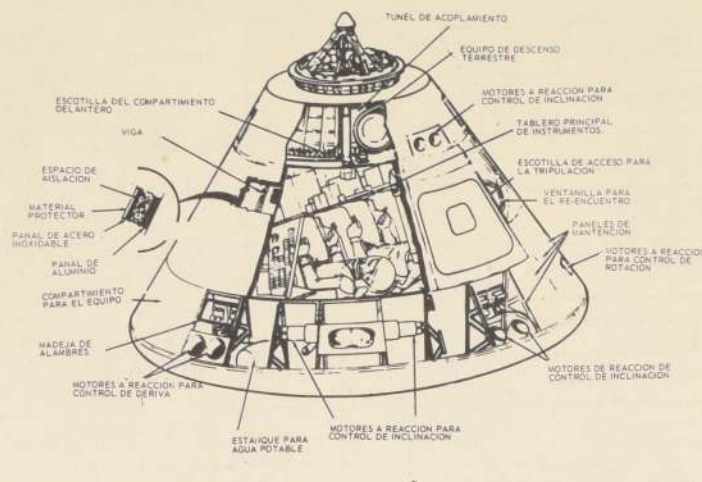
El dibujo en corte muestra el interior del módulo de comando de la Apollo 11, en el que tres astronautas regresarán a la Tierra una vez cumplida su misión en la Luna.
