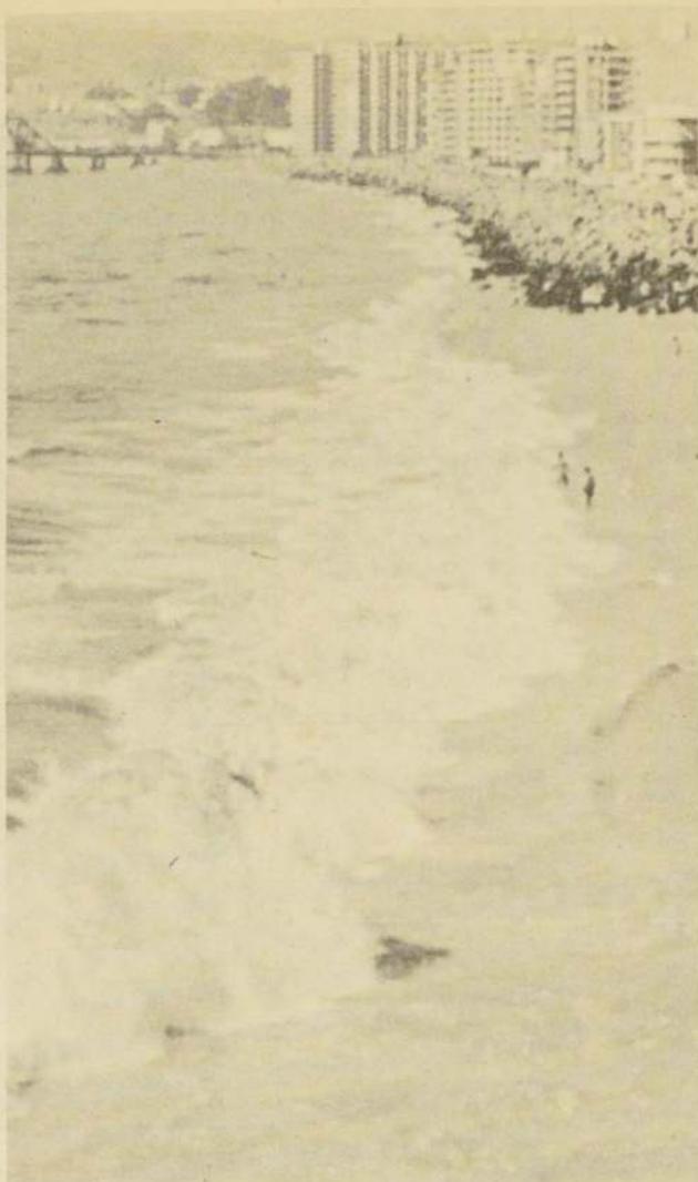
Una corriente cálida del Pacífico es la causa de la marea roja en el litoral porteño, afirmó el oceanólogo de la Universidad de Chile, Eduardo Reyes.
