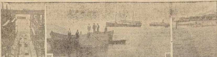
De izquierda a derecha: 1. Uno de los varaderos. — 2. El fondeamiento del primer cajón. — 3. Tres cajones fondeados.
