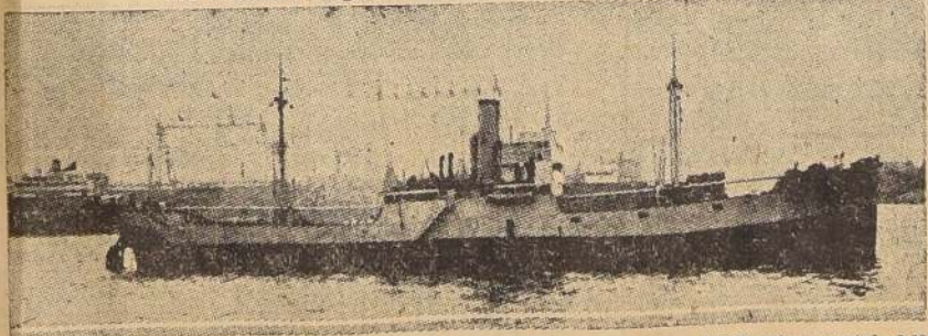
El transporte "VALDIVIA". — Características: eslora, 89 metros; manga, 12,30 mts.; puntal, 6,50 metros; 3,000 toneladas. Motor de triple expansión.
