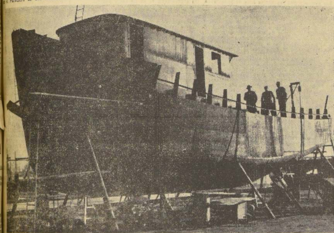
ES "GILDA" — Este es el primer barco pesquero de acero, construido en Chile. Lo hizo "Maestranza Maipú", con un diseño del famoso arquitecto naval de los Estados Unidos, H. C. Hanson. "Gilda" (fue bautizada por su dueña, la "Pesquera Humboldt"), viajará por tierra desde Maipú hasta San Antonio. En el grabado, los altos jefes de la Maestranza inspeccionan la obra, que quedará totalmente terminada a fines de septiembre.
