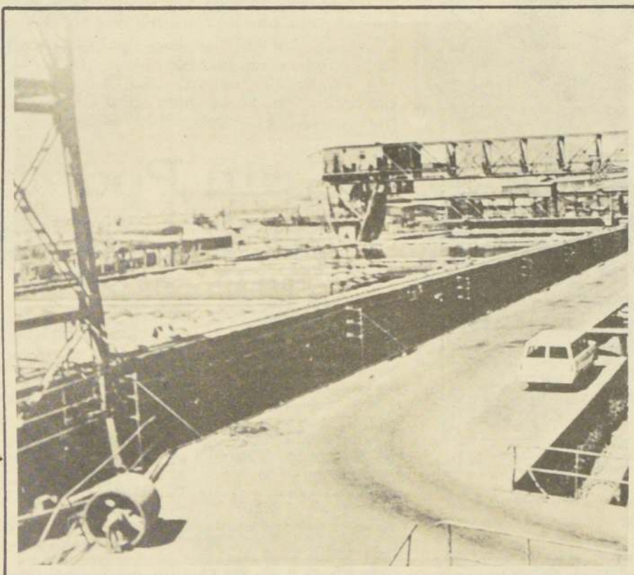
LIXIVIACION.— Instalaciones de una de las plantas de Lixiviación de cobre, ubicadas en la región de El Loa. Próximamente se construirá una de características similares en la localidad de Tuina, 60 kilómetros al interior de Calama
