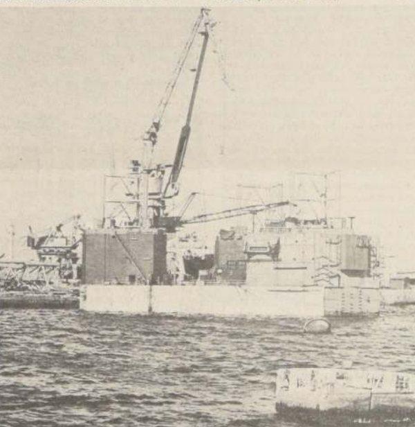
Barco perforador auto-elevatriz "Magallanes" construido en ASMAR para una firma de Estados Unidos destinado a trabajos petroleros en el proyecto Costa Afuera.
