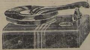
DISCOROLA R-24 B. Motor eléctrico de inducción; corriente alterna; pick-up con unidad de cristal.
