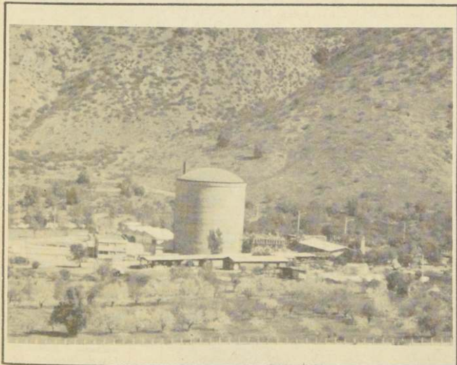
UBICADO A 28 KMS. DE SANTIAGO, el reactor nuclear experimental de Lo Aguirre tiene una potencia de 20 MW.
