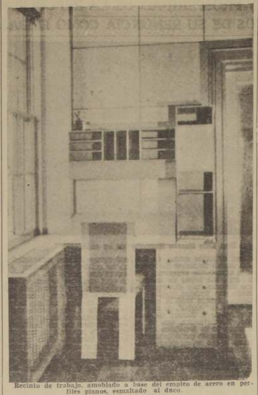
Recinto de trabajo, amueblado a base del empleo de acero en perfiles planos, esmaltado al frío.
