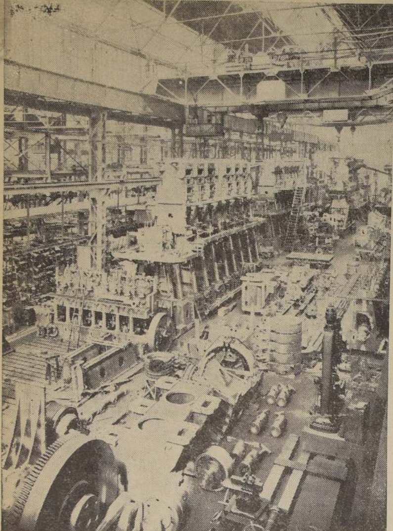
Vista parcial del taller de montaje de Motores DIESEL de gran potencia, actualmente de Deweka (antes Astilleros Imperiales)
