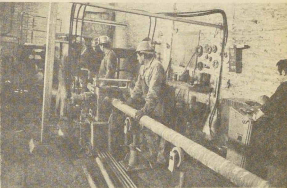
La prensa horizontal con trefiladora y la fundición continua horizontal, departamentos vitales en la firma KAMET, que además cuenta con un completo laboratorio para el control de calidad.
