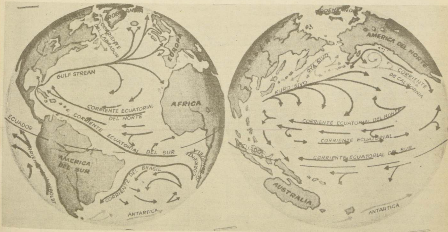
Representación de sistema de Corrientes Marinas. La representación permite apreciar su orientación como factores modificadores del clima.
