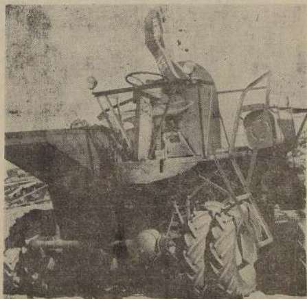
Una de las modernas cosechadoras automáticas del Servicio de Equipos Agrícolas Mecanizados. Con 180 máquinas iguales a ésta, ha sido posible cosechar hasta la fecha más de 41 mil hectáreas de cereales.
