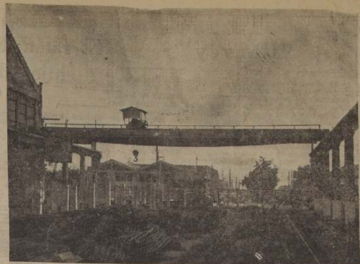
PUENTE GRUA PARA MAESTRANZA DE SAN BERNARDO. — Durante la fiesta realizada ayer en la Maestranza de San Bernardo, con asistencia de S. E. el Presidente de la República, se efectuó la inauguración de un puente rodante para grúa de 15 toneladas construido para esa maestranza por "Socometal".— El puente rodante para grúa fue construido totalmente de planchas dobladas y soldados al arco eléctrico. Sus características, son: Luz (distancia entre eje de rieles) 23.45 mts.; longitud máxima del puente 23.79 mts.; Ancho máximo del puente 4.56 mts.; altura de la viga al centro, (incluso riel), 1.32 mts.; potencia del motor de tracción 36 HP. y velocidad de tracción cargado 2 metros. En el grabado, un aspecto del puente rodante, cuya construcción e instalación ha constituido un nuevo triunfo para "Socometal" y sus técnicos.
