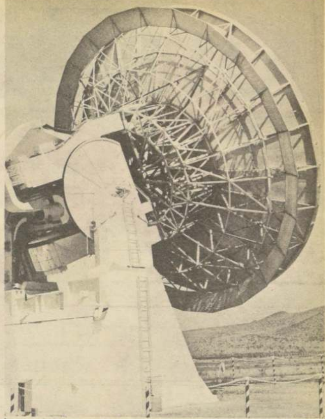
Antena de la estación de rastreo que tiene la NASA y la U. de Chile en la localidad de Peldehue. Durante 20 años han recibido vital información.
