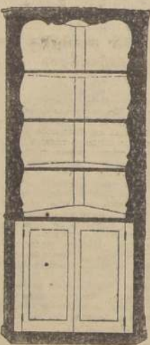
Para un pequeño comedor es indispensable este esquinero en forma de estante y armario. Su construcción es sencillísima y no lleva más adorno que el pequeño filete que hace marco a la parte superior.
