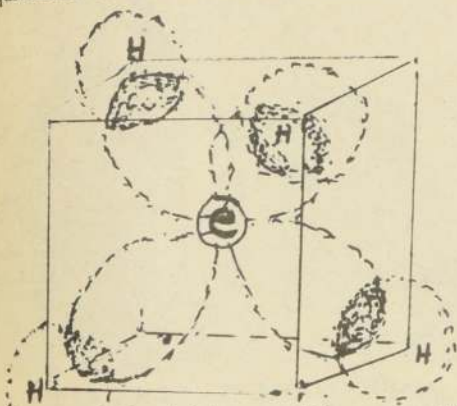
En el enlace participan un orbital S y 3 orbitales P. O sea \text{Sp}^3 . La estructura de la molécula \text{CH}_4 es tetraédrica con ángulos de 109^\circ 28'
