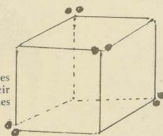
En el enlace participan un orbital S y 3 orbitales P. O sea \text{Sp}^3 . La estructura de la molécula \text{CH}_4 es tetraédrica con ángulos de 109^\circ 28'
