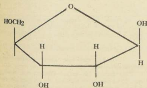
Estructura química de la ribosa
