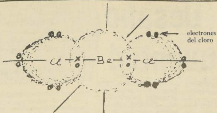
Estructura lineal de la Molécula \text{BeCl}_2 con ángulos \text{Be-Cl} de 180^\circ
