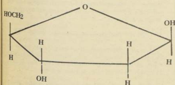
Estructura química de desoxiribosa
