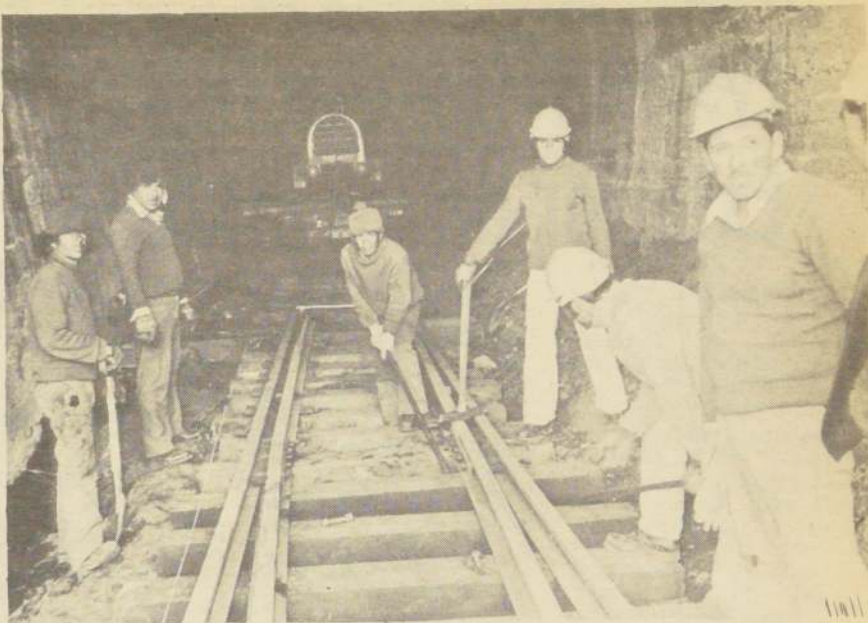
Faenas en el interior del Túnel ferroviario internacional Caracoles-Las Cuevas. El 20 de éste mes está prevista la finalización y su construcción significó 3.089.723 pesos.
