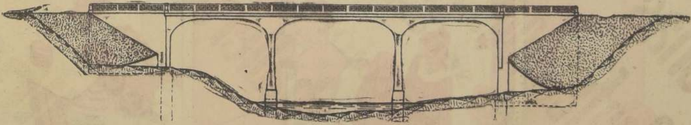
PUENTE LLO-LLEO, EN LLO-LLEO; de concreto armado. Marco rígido de tres tra-
