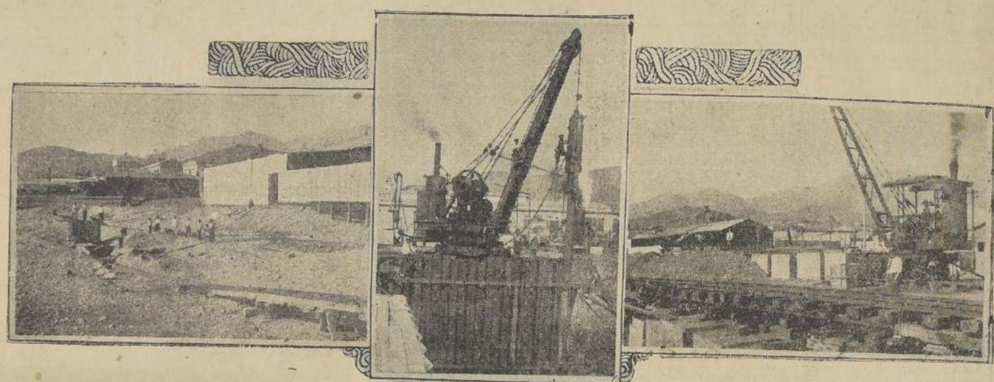
1.—Recopilación de ripio para rellenar el terraplén del antiguo malecón.—2. Martinete a vapor que sirve para plantar las tablas de hierro especial; miden 10 metros de largo; 5 mts. van enterrados y 5 en la superficie. Esta muralla tendrá 100 metros de largo.—3. Grúa que sube los carros de ripio para el relleno.
