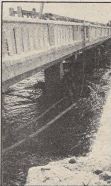
Personal de Vialidad procederá a sacar el puente ACROW que sirvió de alternativa de tránsito por el estero Conchalí.
