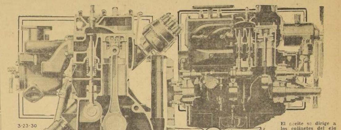
Sección de un motor de ocho cilindros en línea, que se ha anunciado recientemente.
