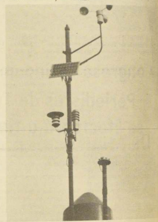
EN LA ALTA CORDILLERA la plataforma está enterrada bajo la nieve y permanecen en la superficie sólo los sensores y la antena.
