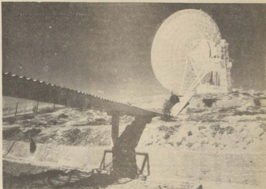
Antena parabólica del radar de rastreo de la Estación Terrestre de Comunicaciones de Longovillo. Ubicada a pocos kilómetros de Melipilla, esta estación de ENTEL y sus auxiliares permiten el transporte simultáneo de todas las formas de comunicaciones que se requieren: telefonía, telegrafía, teletipografía, radiodifusión, televisión y telecomandos.
