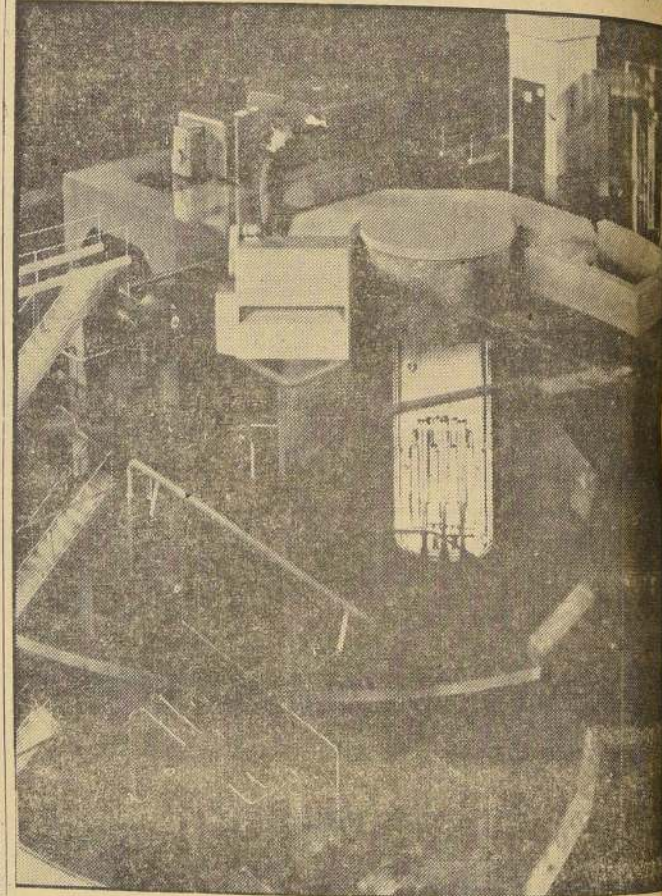
HE AQUI un corte que revela intimidades del reactor de investigación, perteneciente al Laboratorio Nacional de Argonne, EE. UU. Se trata de un reactor de agua pesada, derivado y refrigerado, construido en 1953. La sección en corte muestra el conjunto de elementos combustibles productores de uranio, y las instalaciones experimentales.
