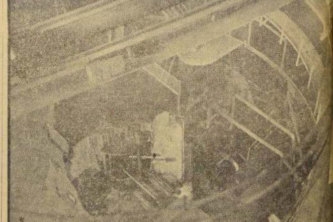
3 PORCION CORRESPONDIENTE al reactor, propiamente tal, del Reactor Experimental de Agua Hirviendo del Laboratorio de Argonne. La cámara de presión, que se presenta en corte, contiene elementos combustibles productores de uranio, con varillas de control que absorben los neutrones. El vapor generado en la cámara de presión es enviado por un separador a la turbina que se ve en la parte superior.
