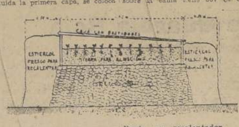
Corte de una cama caliente con recalentador
