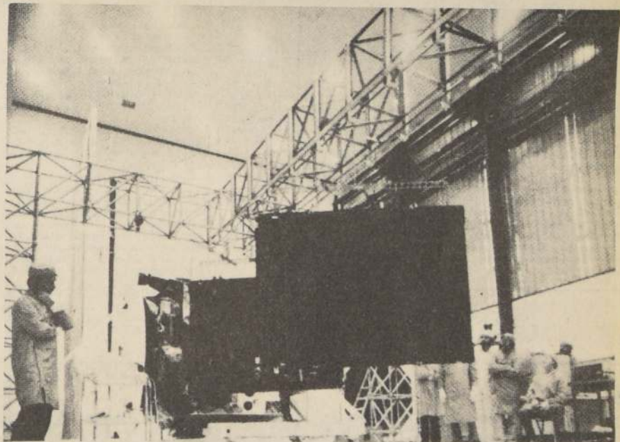
Verificación de las células solares de los paneles del satélite "MARECS A"
