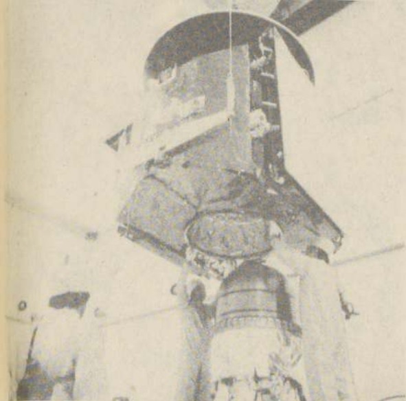
Instalación del satélite "MARECS A" sobre su cabeza de amarre.
