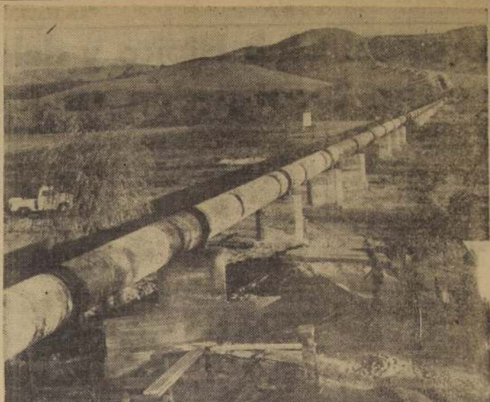
SIFON LIMACHE. VALPARAISO. — El grabado muestra el sifón de acero más grande de Chile. Fue fabricado e instalado por la Maestranza "Maipú", para la aducción de agua potable desde Las Vegas a Valparaíso. Tiene 4.800 metros de largo; un metro 40 centímetros de diámetro, y trabaja a una presión de 180 metros de columna de agua. Las obras fueron visitadas el martes por el Ministro de Obras Públicas, señor Pablo Pérez Zañartu, y se informó que Valparaíso tendrá agua potable de Las Vegas a fines del presente año.
