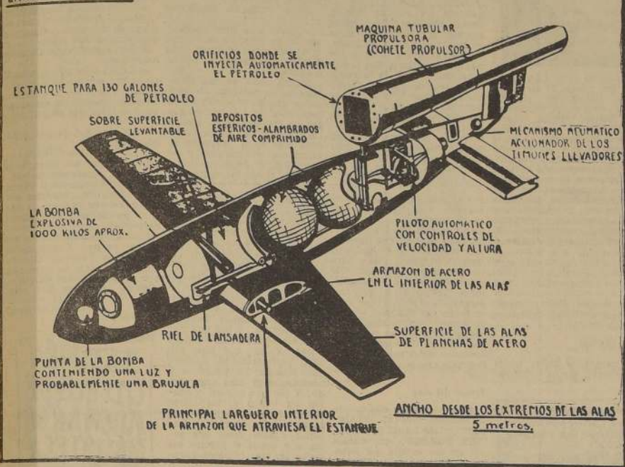
DIAGRAMA DE UN AVION - COHETE
