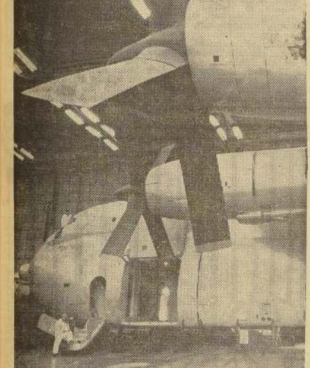
EL PODEROSO DOUGLAS C-132 TENDRA "16" RUEDAS. — La Douglas Aircraft Company lanzará dentro de poco su poderoso Douglas C-132, cuyas inmensas hélices de cuatro aspas serán movidas por turbo-motores que desarrollarán 15.000 caballos de fuerza cada uno. El tren de aterrizaje principal tendrá 16 ruedas, dispuestas en dos unidades cuadruples y coxiales a cada lado del fuselaje y un juego doble en la nariz. Su alto poder de despegue, más su exclusivo tren de aterrizaje, permitirá el gigantesco aparato operar desde pistas comunes y corrientes. El Douglas C-132 representa los más nuevos conceptos de transporte y abastecimiento desplegados por la Fuerza Aérea de los Estados Unidos.
