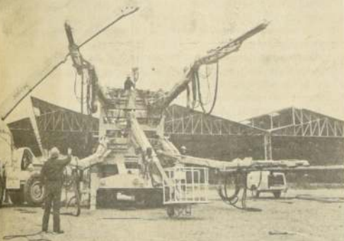
El Promec T-213 de Atlas Copco vuelve a participar activamente en el progreso de Chile, esta vez en la construcción del Complejo Hidroeléctrico Colbún-Machicura. Dos unidades de esta máquina se reacondicionaron en el país por Atlas Copco Chile.
