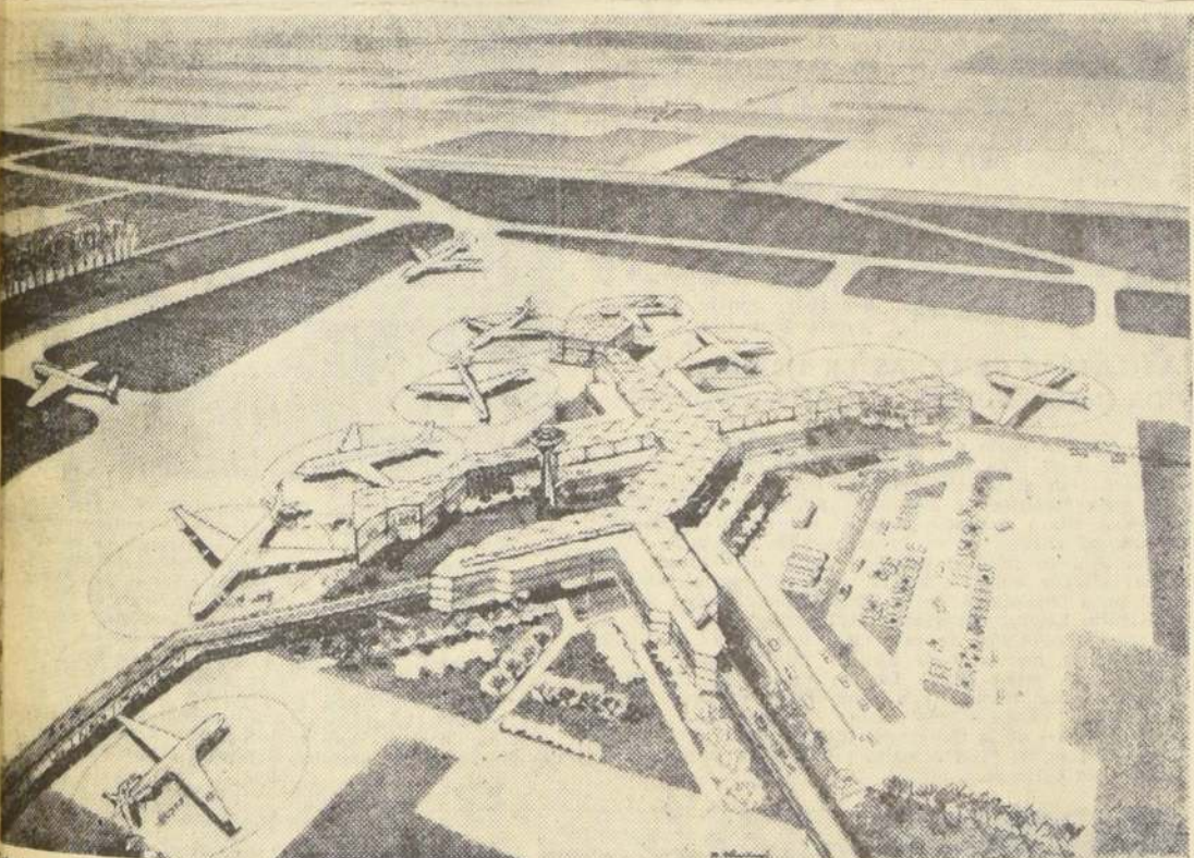
Esta "maqueta" muestra lo que será el futuro aeródromo de Pudahuel, para cuya construcción el Fondo de Préstamos de Desarrollo otorgó a Chile un crédito de 10 millones 500 mil dólares. Será puesto en servicio en 1962. Esta maqueta muestra el arribo de modernas máquinas de retroimpulso y la ubicación simultánea de 38 aviones. Los planes del moderno aeropuerto fueron encomendados a la Alirva Engineering Corporation y los arquitectos chilenos Jaime Larraín, Oscar Larraín y Roberto Müller. Pudahuel estará unido directamente con Valparaíso y Santiago, y en su construcción se empleará exclusivamente personal y material nacionales.
