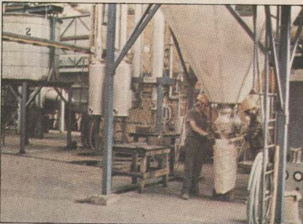
En las instalaciones de su planta en Escuadrón la Soc. Nacional de Tanino, con tecnología desarrollada por CIDERE-Biobío, está produciendo parte de los requerimientos de tanino para la industria chilena de curtiduría.
