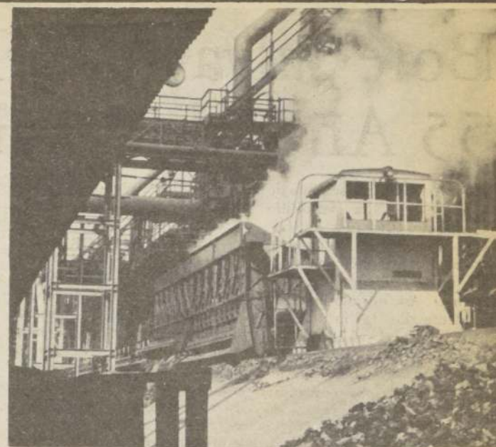
Planta de Coque de Huachipato, unidad que cumplió 30 años en operación.
