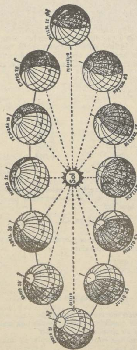
Fig. 9.—La Tierra en sus doce posiciones anuales sobre la eclíptica. Si bien se observa, se verá que en todas estas posiciones el eje de la Tierra es paralelo a sí mismo y siempre con la misma inclinación con respecto a la eclíptica
