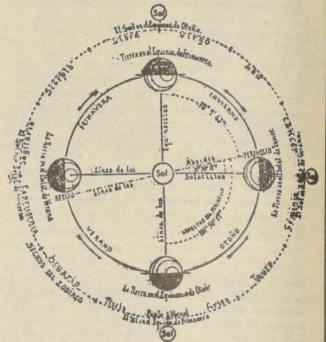
Fig. 5.— Orientación del eje de la Tierra respecto de la eclíptica, con la representación de la longitud del perihelio
