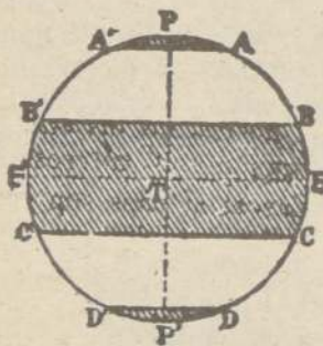
Fig. 3.— Zonas terrestres: CC' BB', zona tórrida; AA' BB' y CC' DD', zonas templadas; APA y DP'D', zonas glaciales
