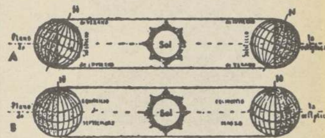
Fig. 10.—A, la Tierra en los solsticios, vista desde el equinoccio de otoño o septiembre; B, la Tierra en los dos equinoccios, vista desde el perihelio o posición de diciembre
