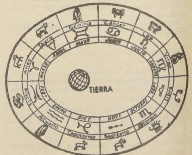
Fig. 6.— Figuras del Zodíaco con sus correspondientes signos
