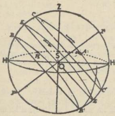
Fig. 7.—Cambios anuales de declinación del Sol
