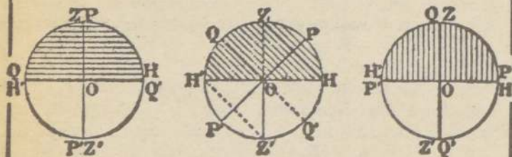
Fig. 4.— Disposición de los paralelos celestes en el polo de la tierra (I); en las zonas templadas (II), y en el Ecuador (III), que da lugar a las llamadas: esferas paralela (I), oblicua (II) y recta (III), y a las distintas zonas climatológicas
