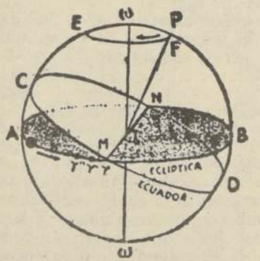
Fig. 8.—Retrogradación del punto vernal (v, v', v'')
