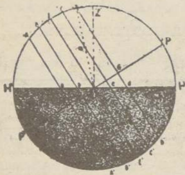
Fig. 2.— Representación gráfica de la duración de los días en las zonas templadas de la Tierra.
