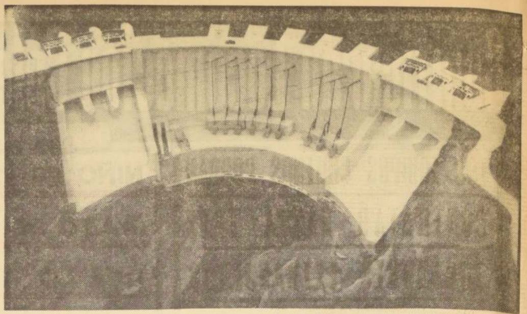
Maquette del proyecto. Aspecto que presentará una vez terminada esta obra monumental de 107 metros de altura, de 300 de largo y con un camino de 9 metros de ancho en la cima. Obsérvense los verederos laterales de emergencia. Esas aguas servirán, entre otros beneficios, para regar una vasta zona de Navidad.
