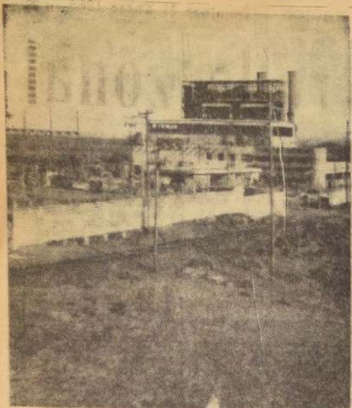
La Planta ENDESA en Huasco, la que con una capacidad de 16.000 Kw. está entregando energía a la zona.
