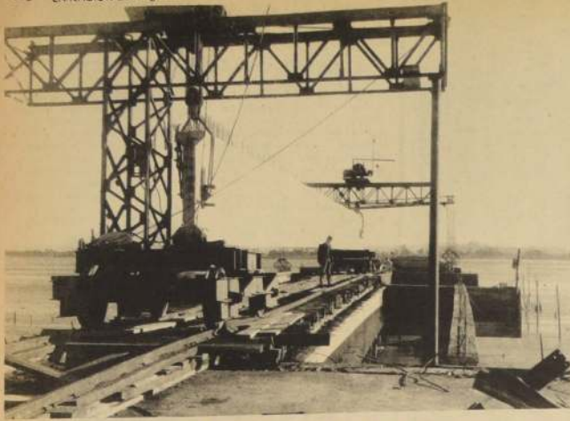
PUENTE BÍO BÍO , en la provincia de Concepción, es el más largo de Chile y uno de los de mayor longitud en Sudamérica. La obra es ejecutada por la Dirección General de Obras Públicas y será inspeccionada por el Ministro Pascual Barraza.
