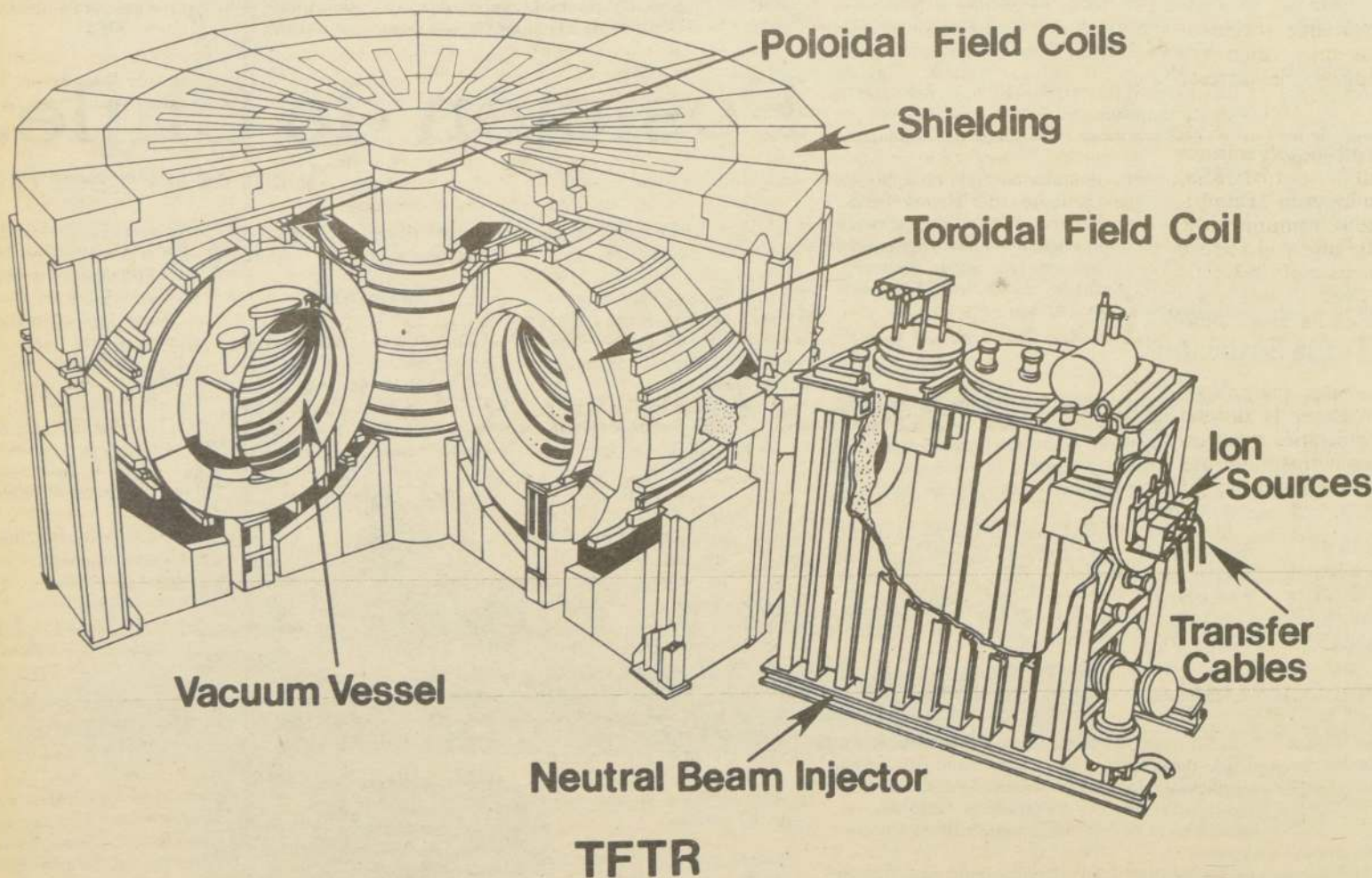
El año próximo comenzará a operar el reactor de fusión de la Universidad de Princeton (EE.UU.), cuyo esquema aparece en el grabado. Se trata de un modelo experimental.
