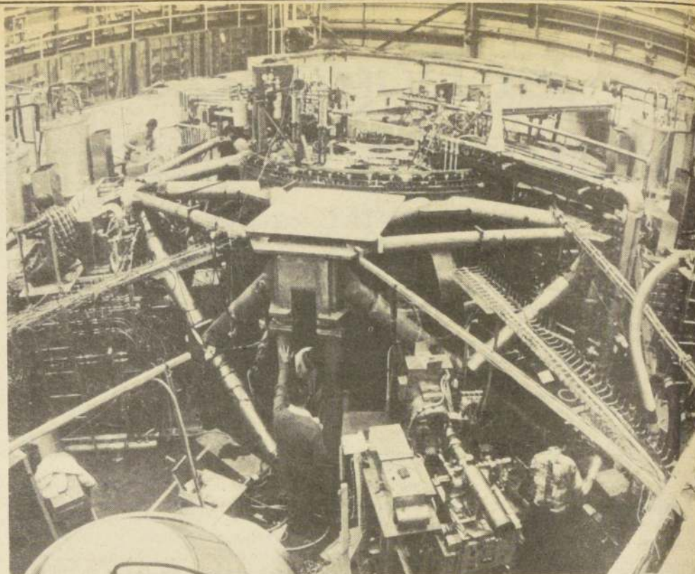
El "Large Torus" de la U. de Princeton es el más grande reactor de fusión nuclear que existe
