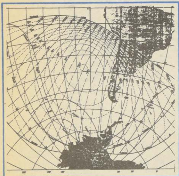
El gráfico muestra la zona que cubrirá el eclipse de Sol del 22 de este mes, desde el Océano Pacífico Austral para terminar en el territorio antártico.
