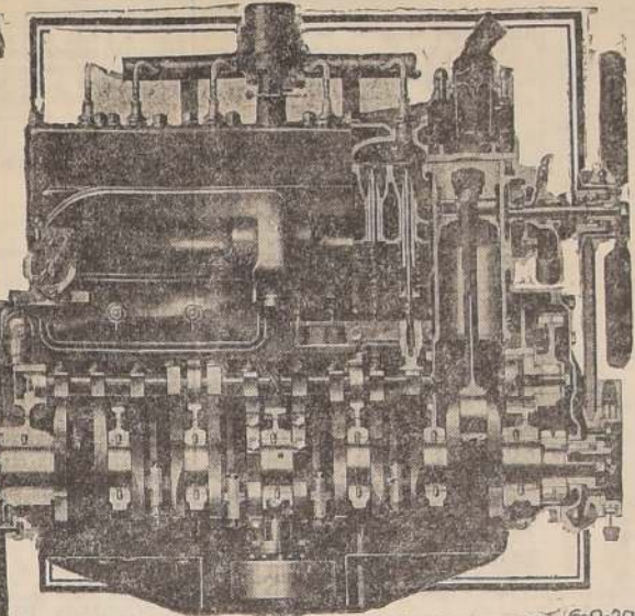
Sección de la parte longitudinal de un motor de alta presión, que muestra las válvulas y las partes del motor que trabajan.
