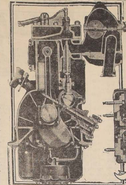
Sección transversal a través de un cilindro de un motor de alta presión, que muestra la cámara de combustión.
