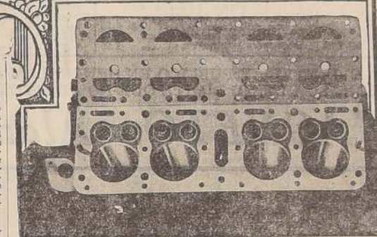
Bloque de cilindros de un automóvil moderno, mostrando los hoyos para la cabeza de los cilindros. Nótese el pulimento de la pieza, que asemeja a un espejo.
