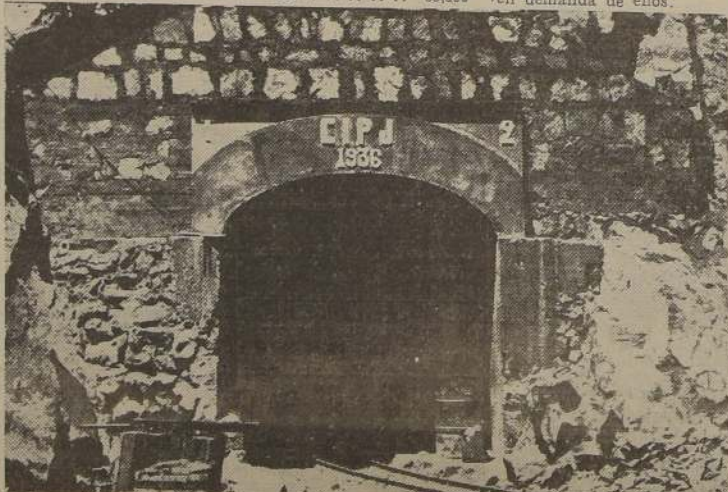
Vista del túnel N.º 2, en las obras de regadío de La Jota, Arequipa. Su capacidad de descarga es de 20 metros cúbicos por segundo, y su longitud total será de 1,400 metros, con un ancho de 3.50 metros. Su altura será de tres metros.
